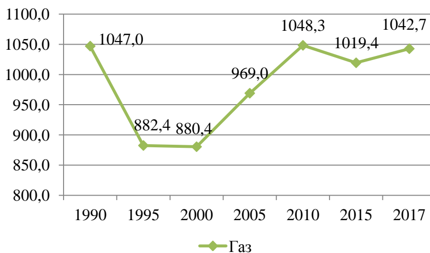
Рисунок 5– Динамика выбросов CO 2 при сжигании газа в странах СНГ, млн т
