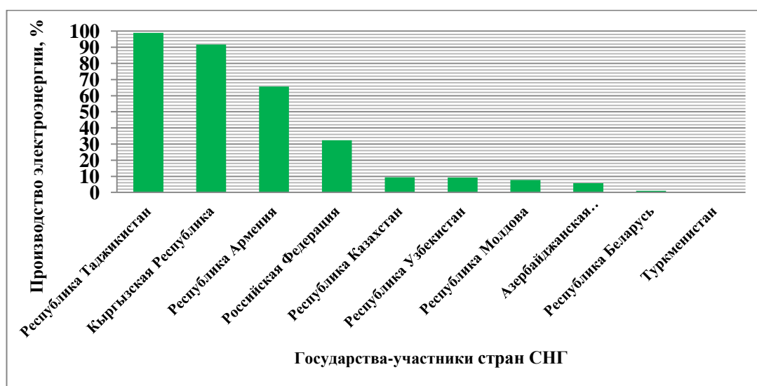
Рисунок 6 – Доля производства электроэнергии на «безуглеродных» источниках энергии (ГЭС, АЭС, ВИЭ) в электроэнергетике стран СНГ, %
