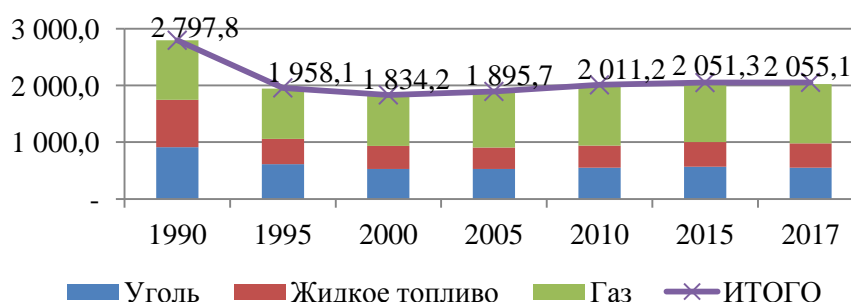
Рисунок 2 – Динамика выбросов CO 2 при сжигании органического топлива в странах СНГ, млн т
